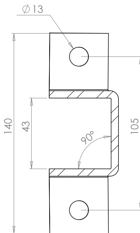
COUPE A-A ECHELLE 1 : 1.5
